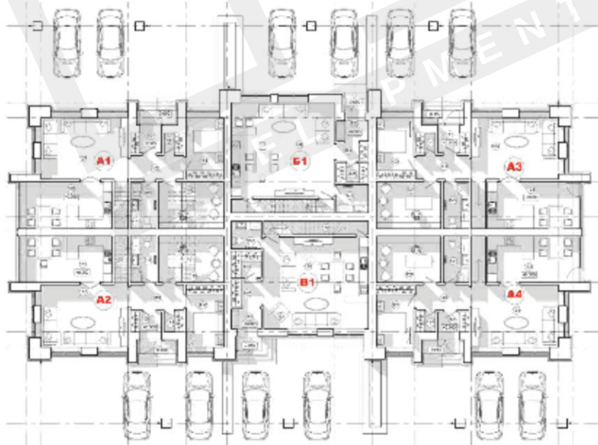
ПРИМЕР ТИПОВОГО ПЛАНА (ДОМ №3)
